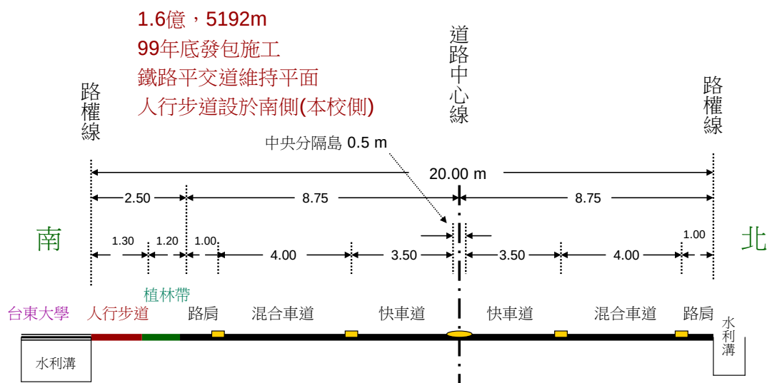
西康路拓寬標準斷面圖
